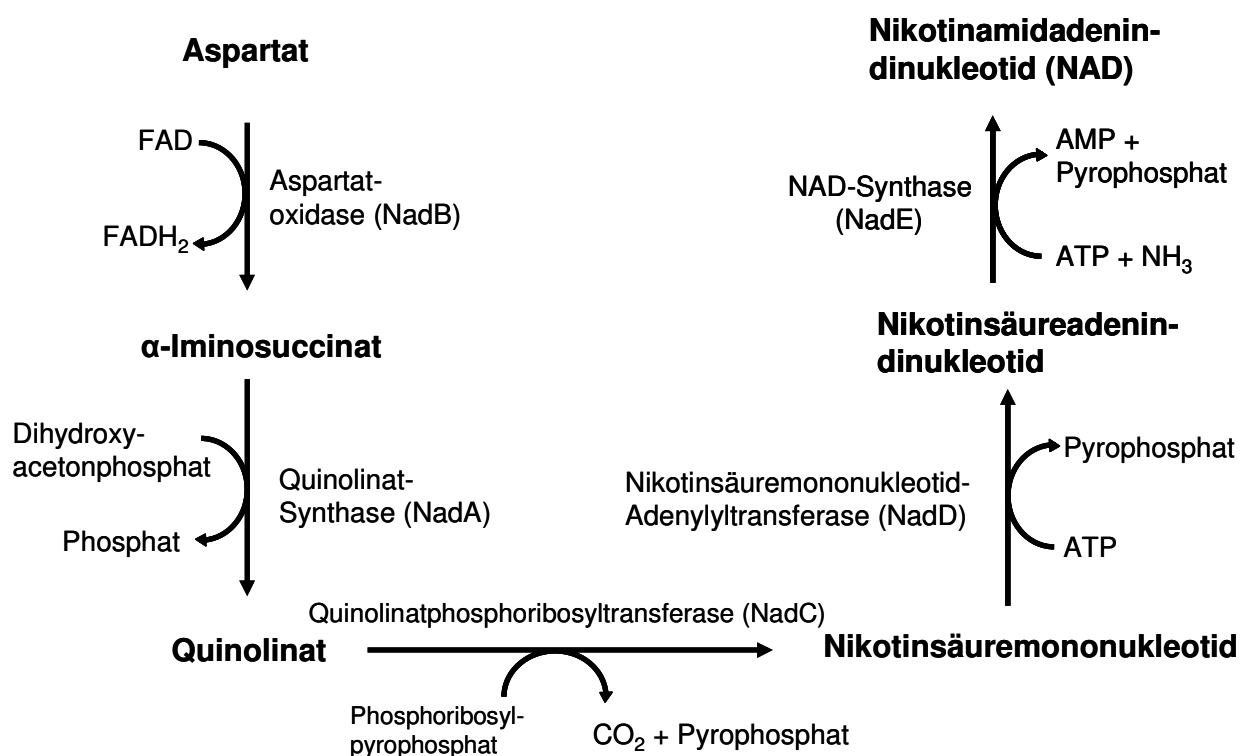
Abb. 2: Stoffwechselweg für die de novo Synthese von NAD in Bakterien.
