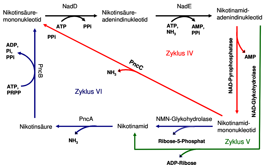
Abb. 3: NAD kann auf vier unterschiedlichen Wegen recycelt werden, Pyridinnukleotidzyklus IV (rot), -zyklus V (grün), -zyklus VI (blau).
